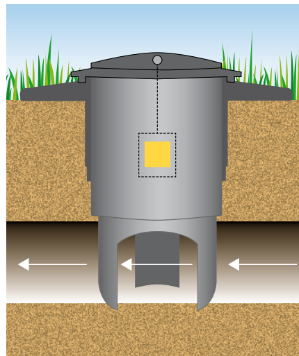
Eingebaute Schermausköderstation
