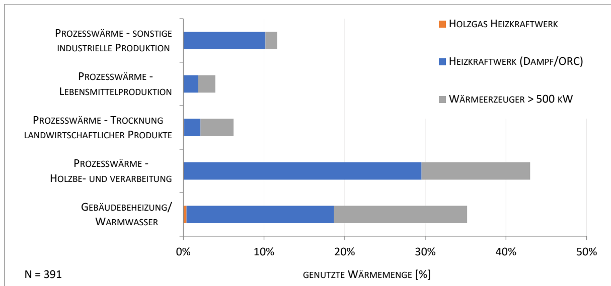
Abbildung 55: Art der Wärmenutzung und deren Anteil an der genutzten Wärmemenge (C.A.R.M.E.N.-Umfrage 2022, Wärmeerzeuger > 500 kW N=296, Heizkraftwerke (Dampf/ORC) N=58, Holzgas Heizkraftwerk N=37).
