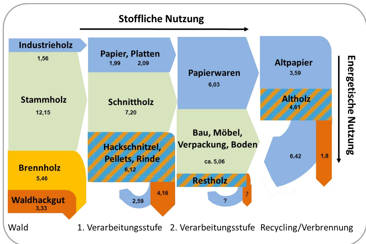
Abbildung 64: Stoffströme der stofflichen und energetischen Holzverwendung in Bayern 2022 in Mio. Fm m. R. bzw. m³.
